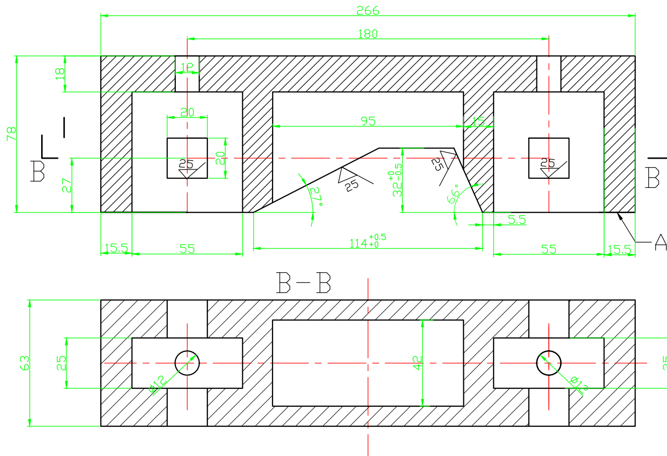
篦冷机固定棒压块
